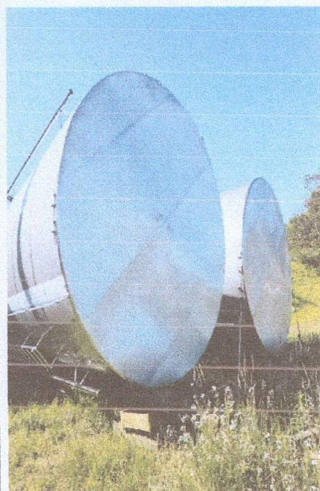
Imagem 6 – Dimensional fundos 3800 mm
