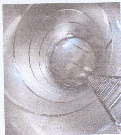
Imagem 2 – Inspeção Visual de Solda e acabamentos internos do Reservatório 02
